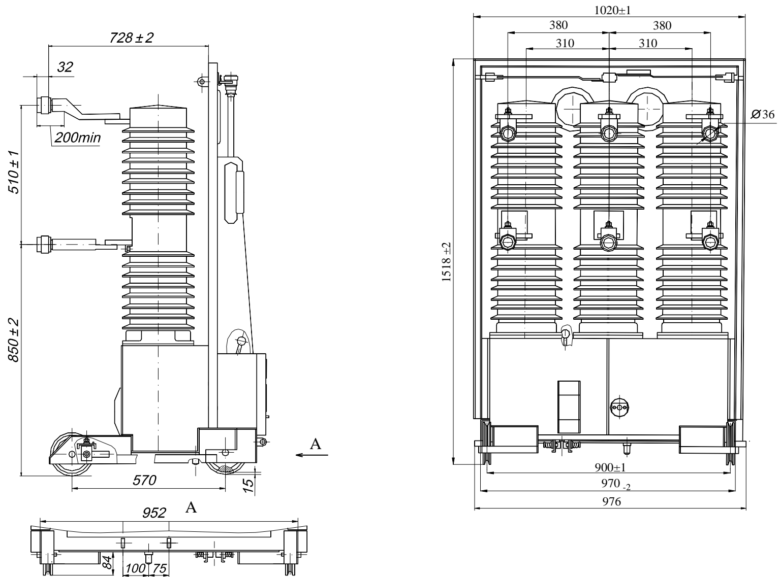
Габаритные, установочные и присоединительные размеры выключателя для шкафа КРУ серии К-35 (вариант ЗАО Петрознергосервис)
