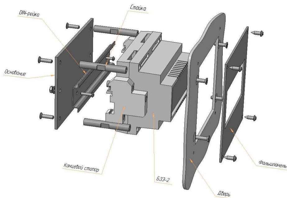
Рисунок Е.2 – Схема установки БЗЭ-2 на двери шкафа
